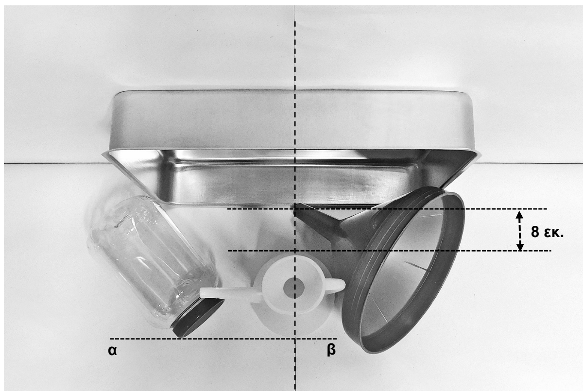
δεύτερη φωτογραφία: κάτοψη
